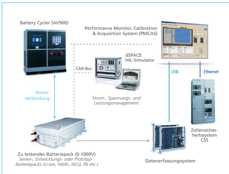
Der Aufbau für den Test der Batteriepacks. Der dSPACE HIL-Simulator ist das Herz des virtuellen Fahrzeugs und simuliert alle für die Tests notwendigen Fahrzeugkomponenten.
